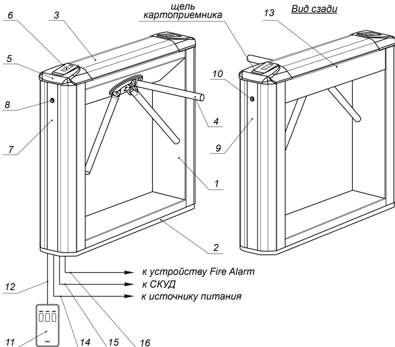
Рисунок 2. Устройство турникета
