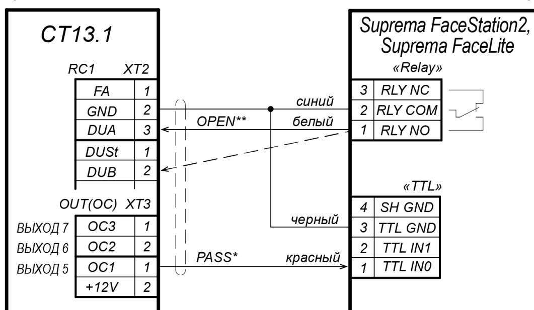
Рисунок 27. Схема подключения ТРЛ производства ZKTeco к контроллеру ЭП
