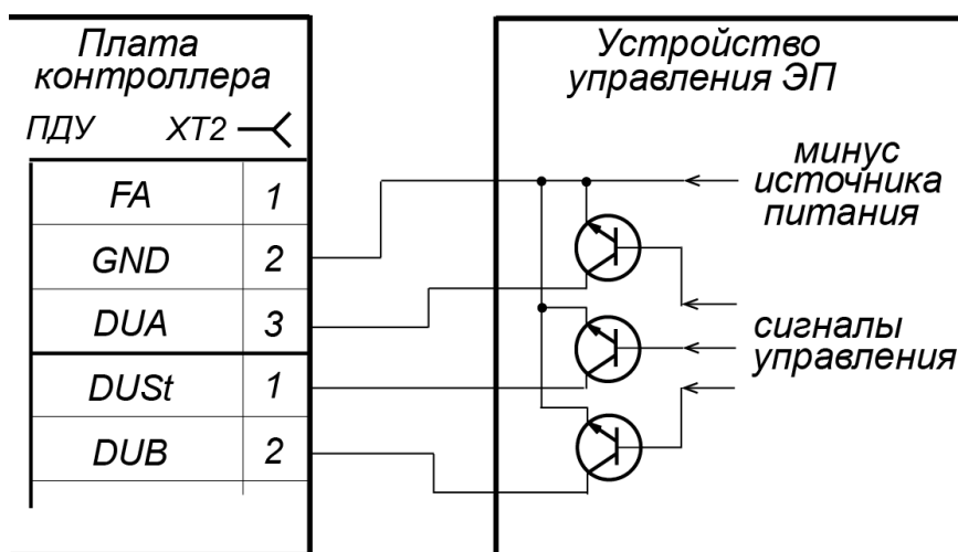
Рисунок 10. Управление ЭП схемой с открытым коллекторным выходом
