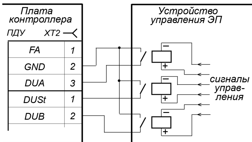
Рисунок 9. Управление ЭП нормально разомкнутым контактом реле
