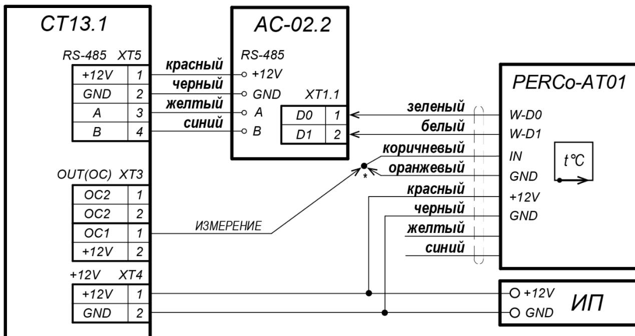
Рисунок 35. Схема подключения к контроллеру ЭП пирометра с конфигурацией «ВВУ с тактированием»
