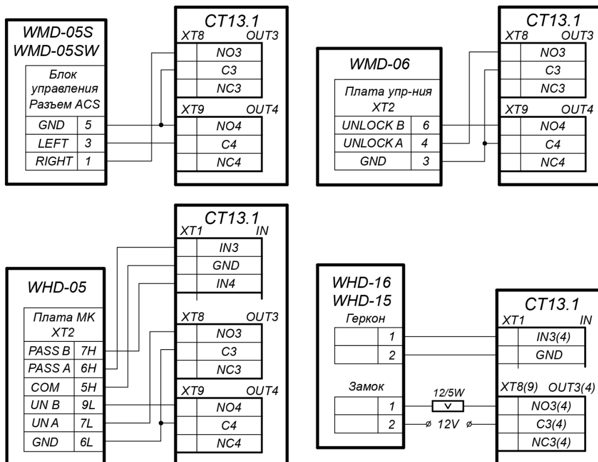
Рисунок 18. Схемы подключений второго ИУ – электромеханической калитки
