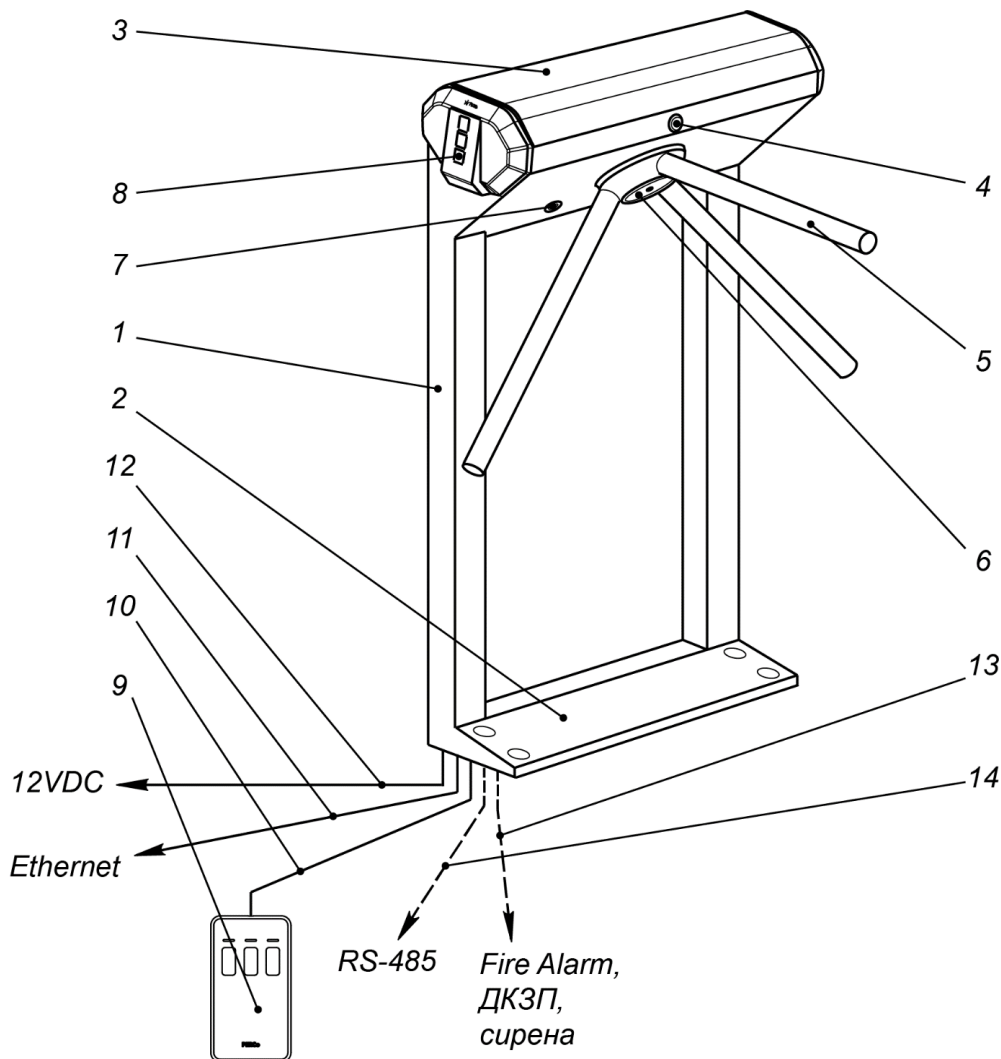
Рисунок 2. Устройство ЭП
