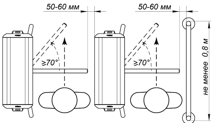
Рисунок 11. Рекомендации по организации зоны прохода
