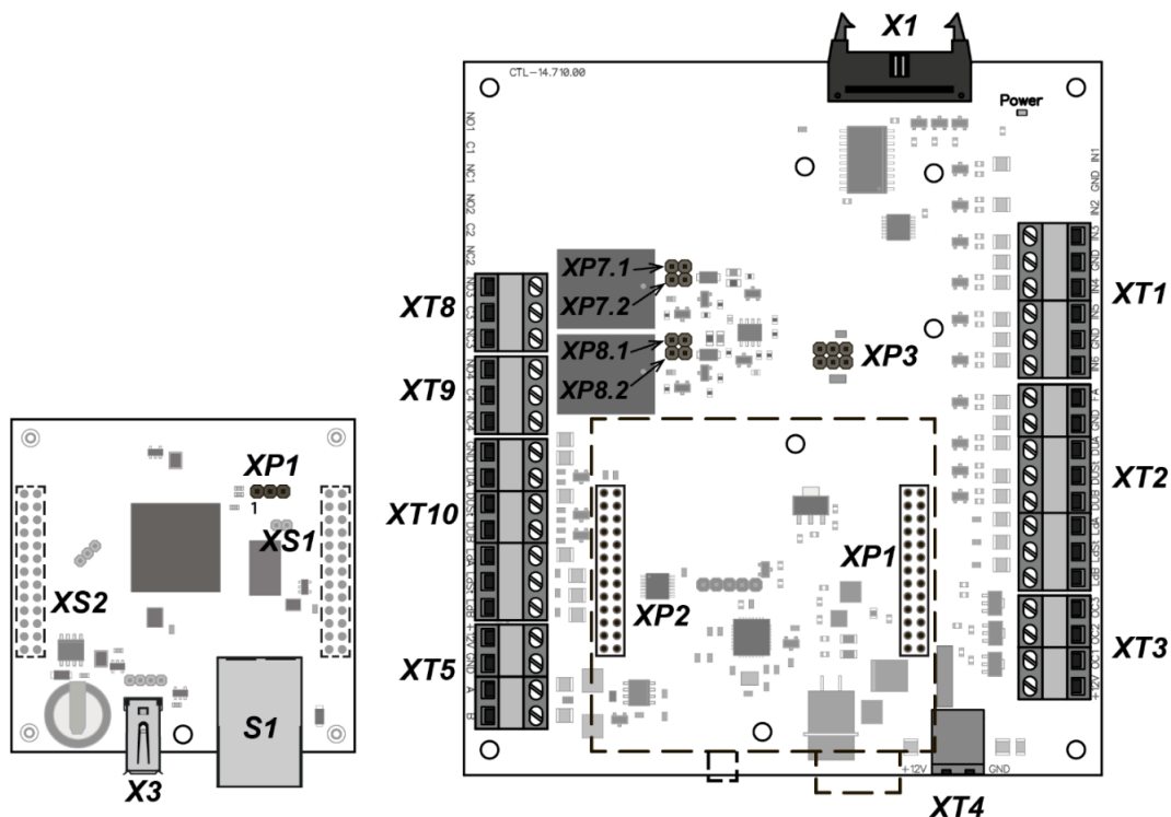
Рисунок 7. Внешний вид верхней и нижней плат контроллера
