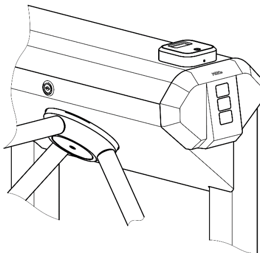
Рисунок 34. Место установки пирометра PERCo-AT01 на крышку ЭП
