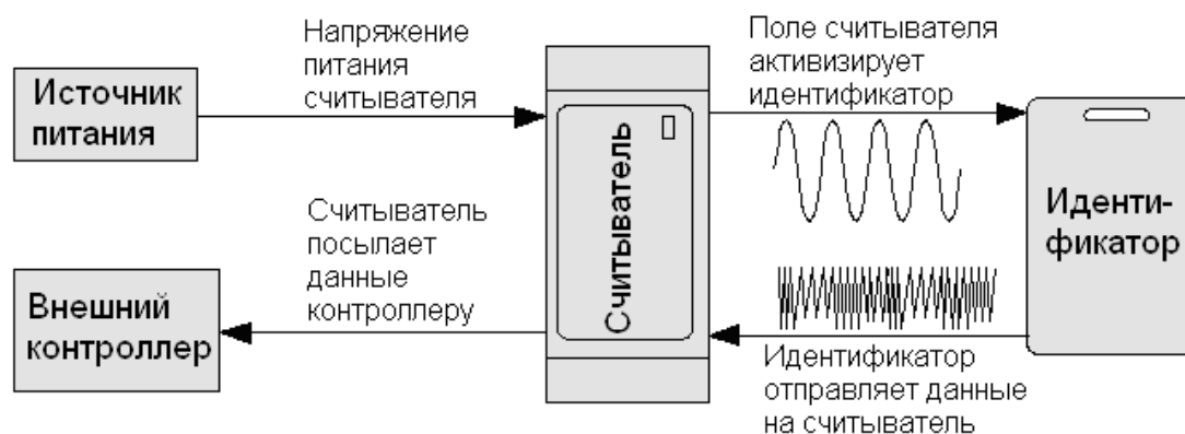
Рисунок 5. Функциональная схема, поясняющая работу считывателя
