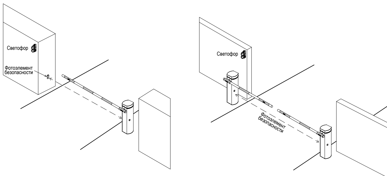
Примеры проектов транспортной проходной с использованием GF03.1
