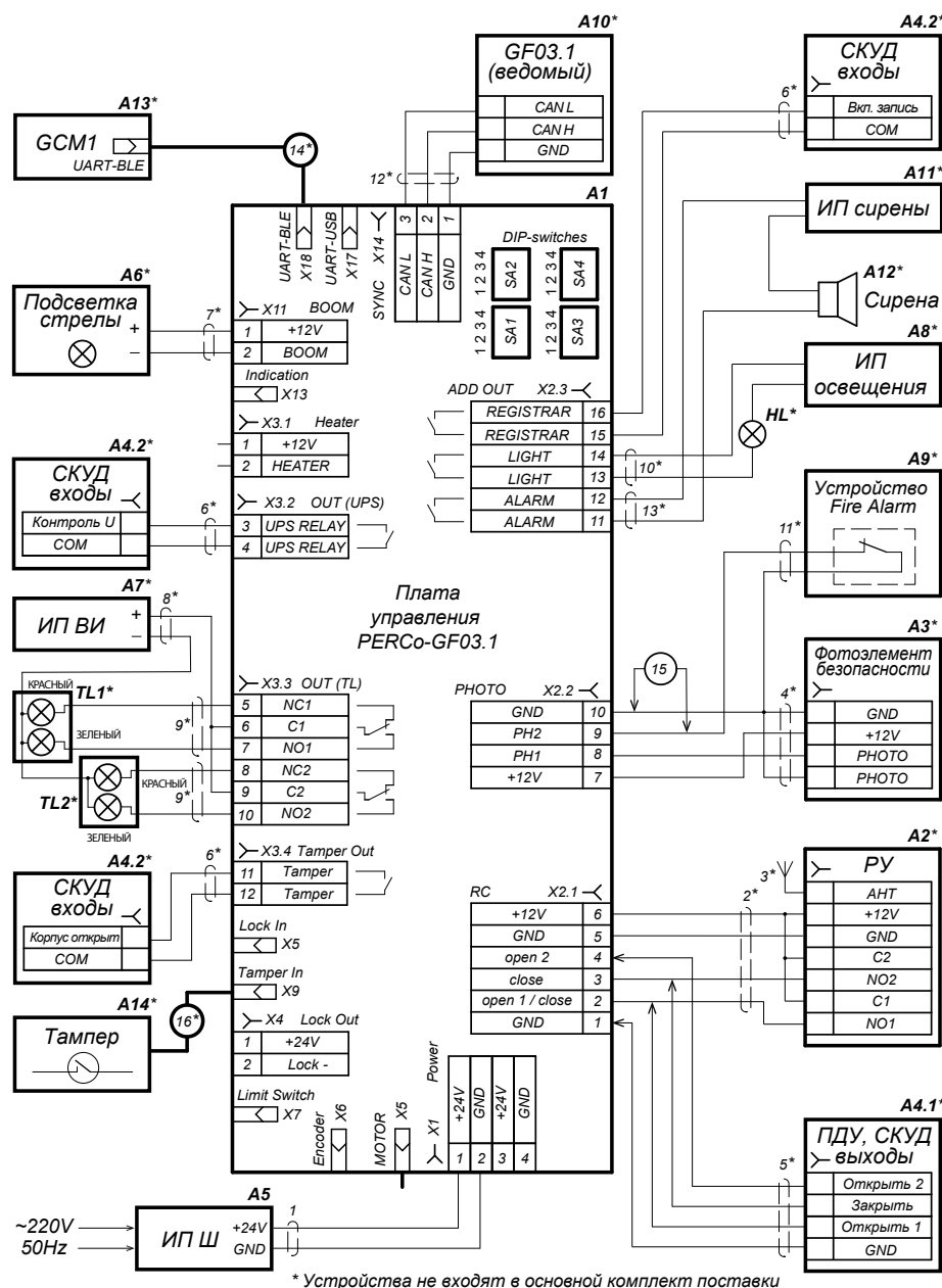
Схема электрических соединений слагбаума GF03.1
