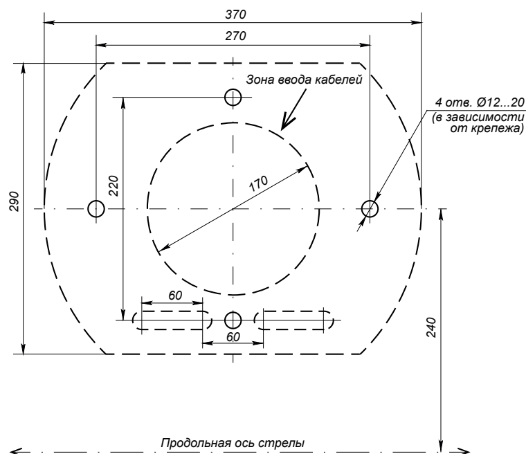
Разметка установочных отверстий шламбаума
