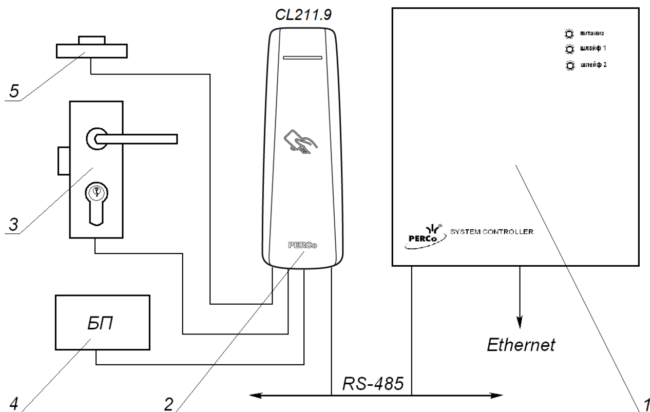
Рисунок 1. Функциональная схема
