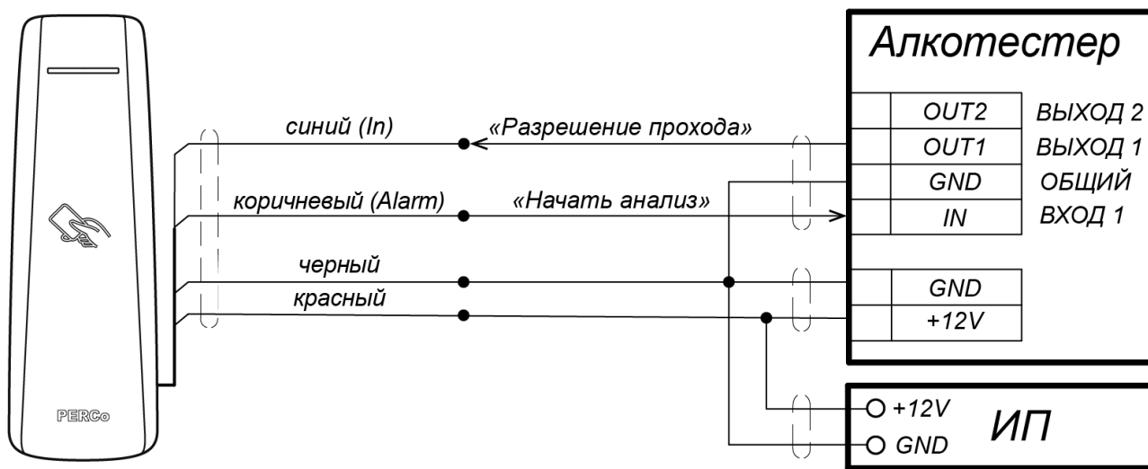
Рисунок 10. Схема подключения ВВУ на примере алкотестера
