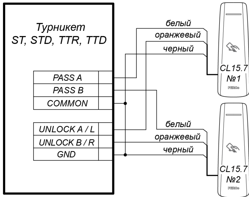
Рисунок 7. Схемы подключений турникетов
