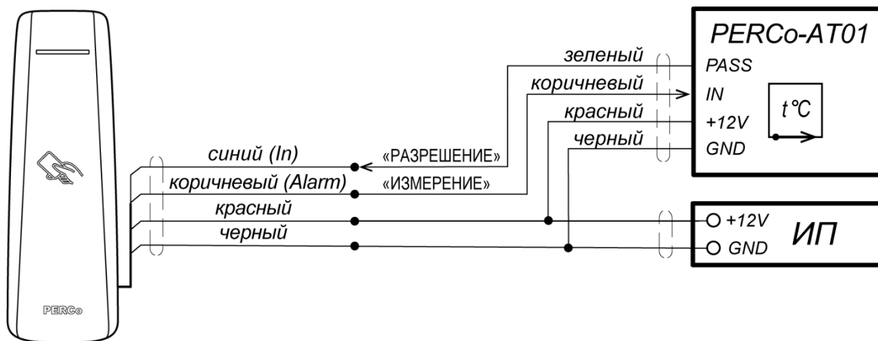
Рисунок 12. Схема подключения пирометра PERCo-AT01 к контроллеру CL15.7
